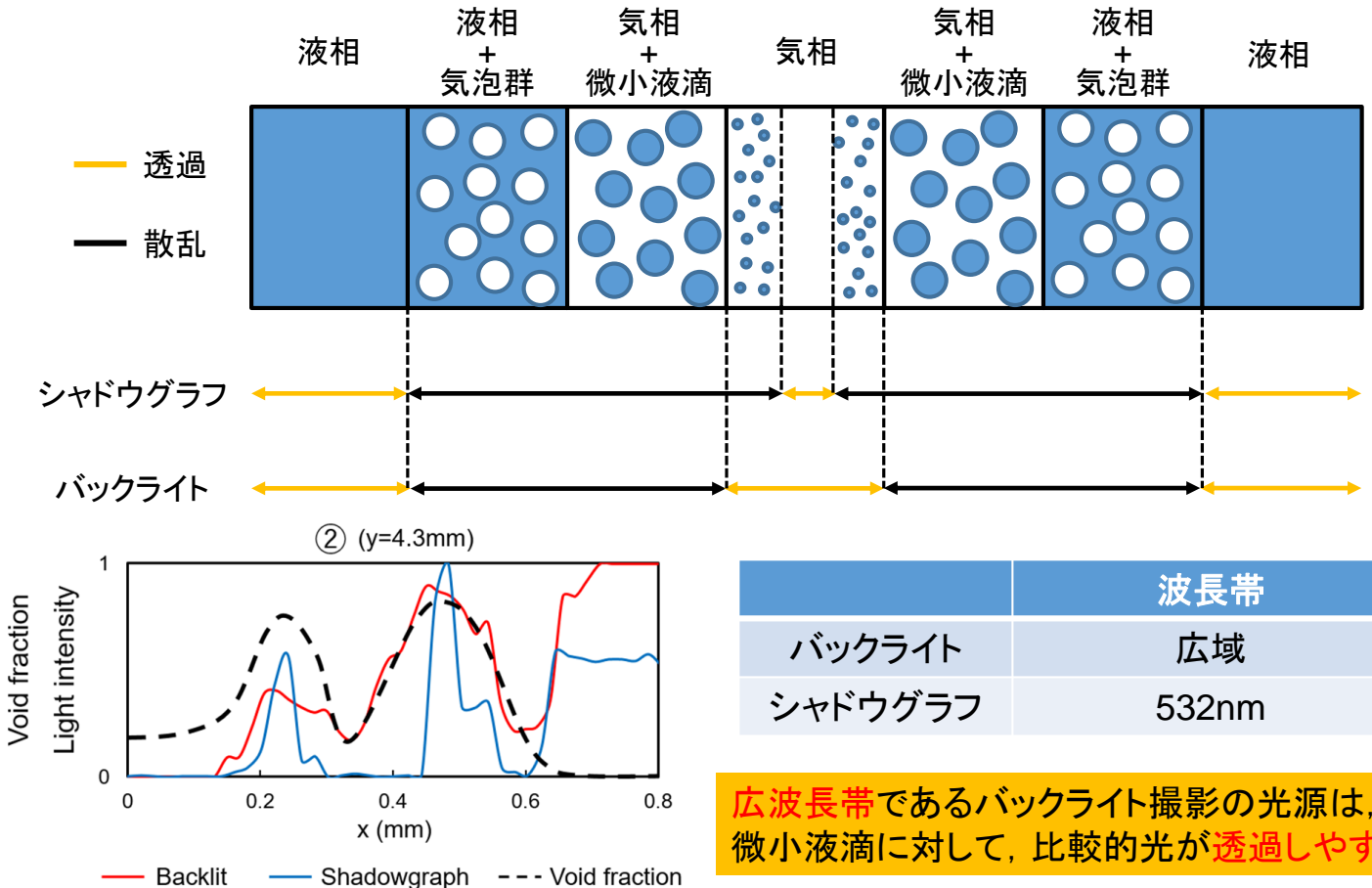
重質油の噴霧におけるノズル内キャビテーションの観察
