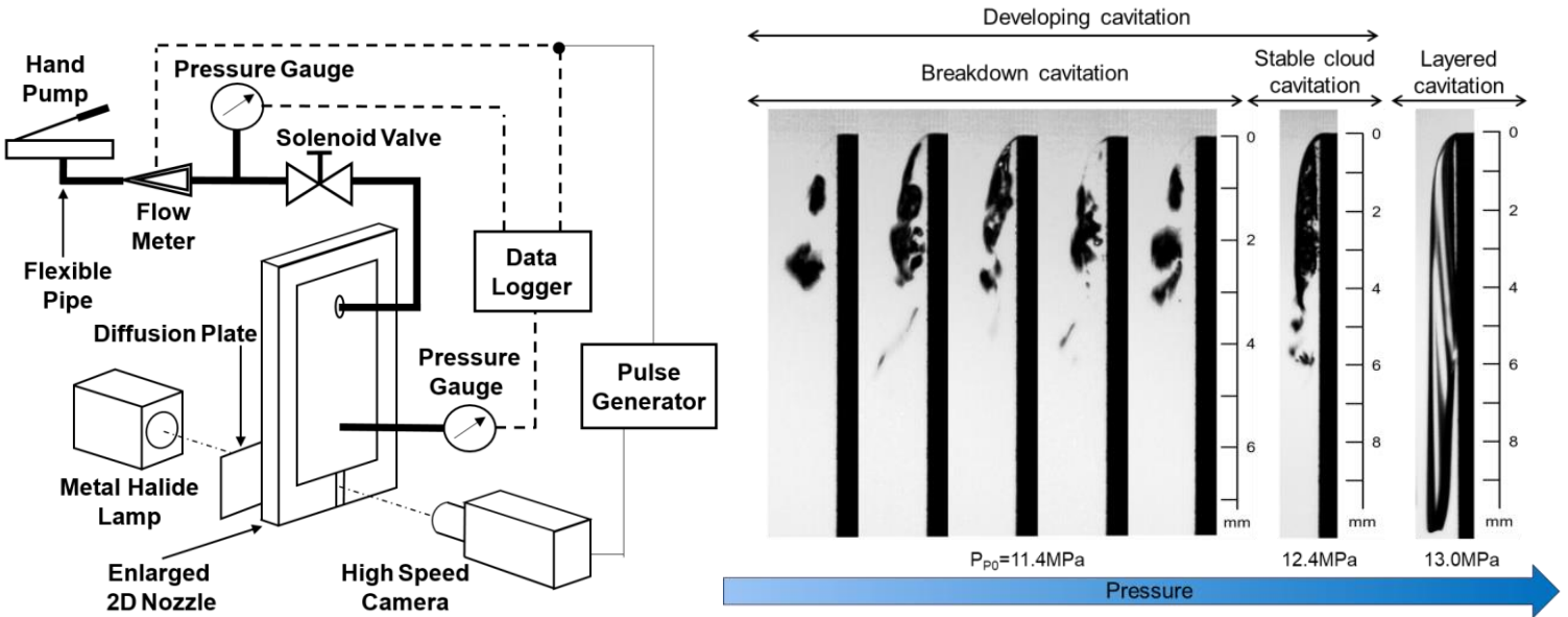
重質油の噴霧におけるノズル内キャビテーションの観察
